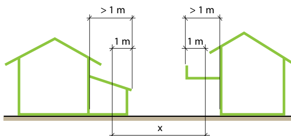
Fig. 6: Voies d'évacuation et issues de secours; zone avec des exigences pour les façades, fenêtres et portes (dessin d'après AEAI)
