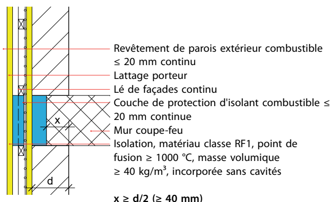
Fig. 7: Revêtement de parois extérieur/couche de protection isolante combustible ≤ 20 mm; raccordement de murs coupe-feu au mur extérieur (dessin d'après AEAI)
