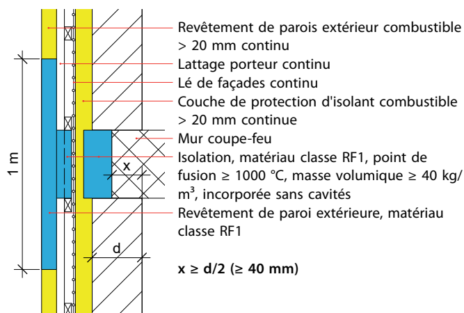
Fig. 8: Revêtement de parois extérieur/couche de protection isolante combustible > 20 mm; raccordement de murs coupe-feu au mur extérieur (dessin d'après AEAI)
