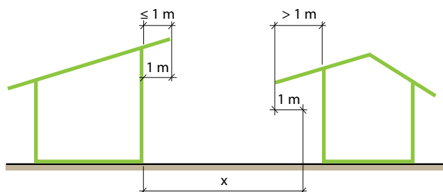
Fig. 5: Distance de protection incendie = x (dessin d'après AEAI)
