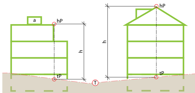
Fig. 4: Géométrie de bâtiment; T = terrain déterminant, h = hauteur totale, tP = point le plus bas sur le terrain déterminant sous la surface de toit, hP = point le plus haut du toit, a = superstructure exigée par la technique (dessin d'après AEAI)
