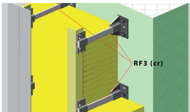
Fig. 3: Fixations ponctuelles
