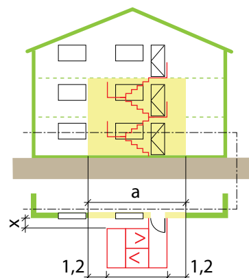
Fig. 6: Voies d'évacuation et issues de secours; zone avec des exigences pour les façades, fenêtres et portes (dessin d'après AEAI)
